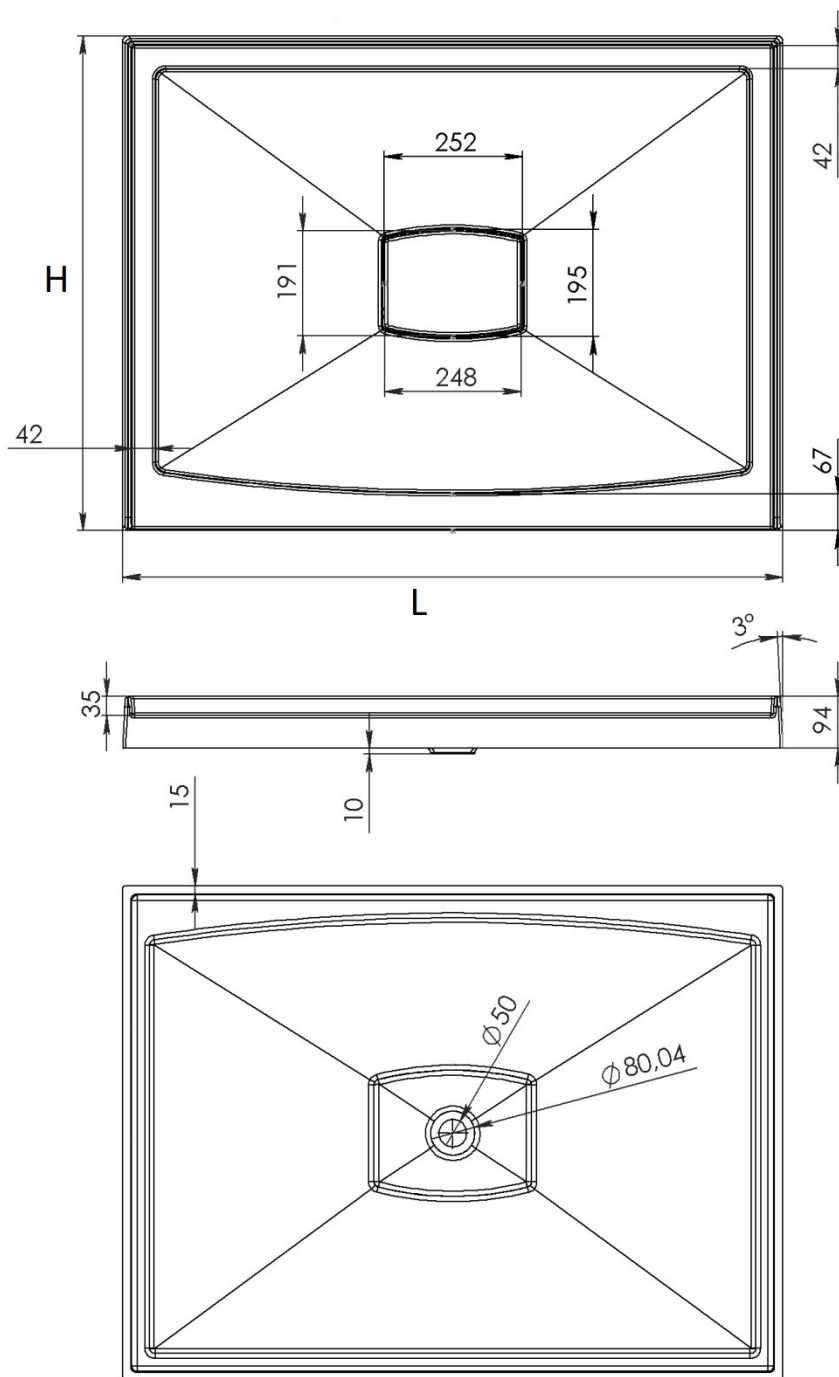
Чертеж: Душевой поддон PESARO маштаб 1:10
